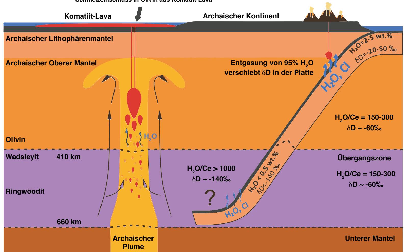
Schmelzeinschluss in Olivin aus Komatiit-Lava
