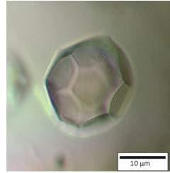
Schmelzeinschluss in Olivin aus Komatiit-Lava
